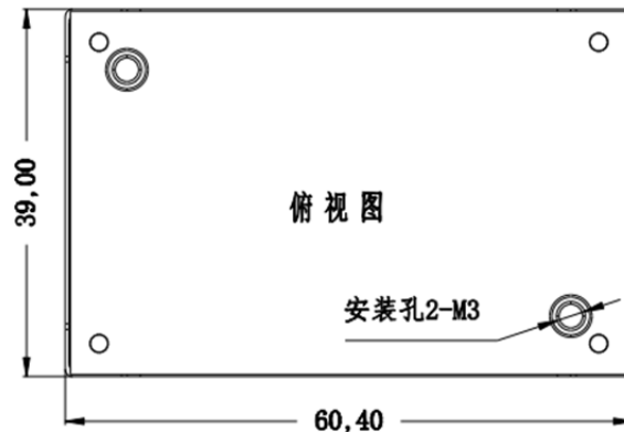
标准型 60.4*39*12.7mm
